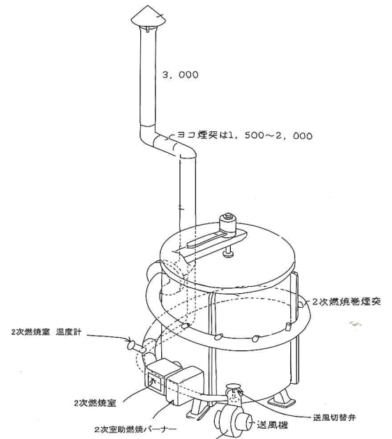
ゴミゼ炉くん CM-20型
