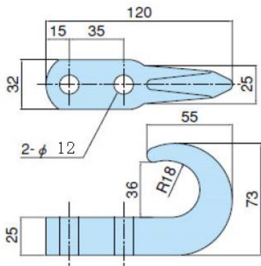
A011580 牽引フック 大型
