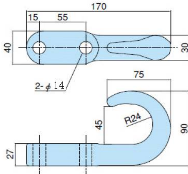
A011570 牽引フック 4ト
