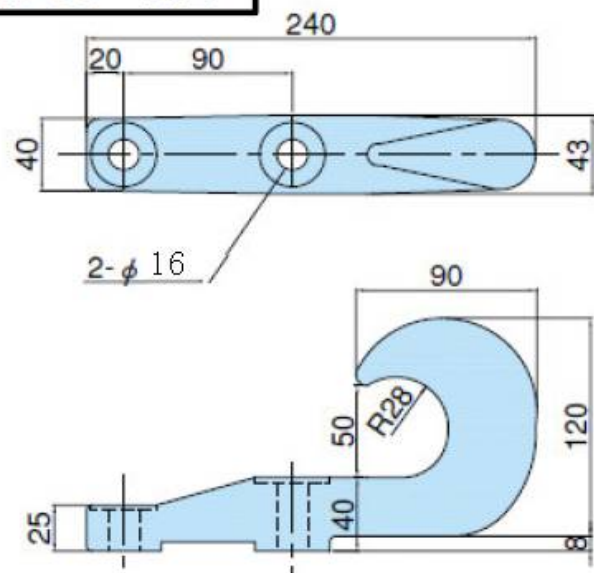
A011580 牽引フック 大型
